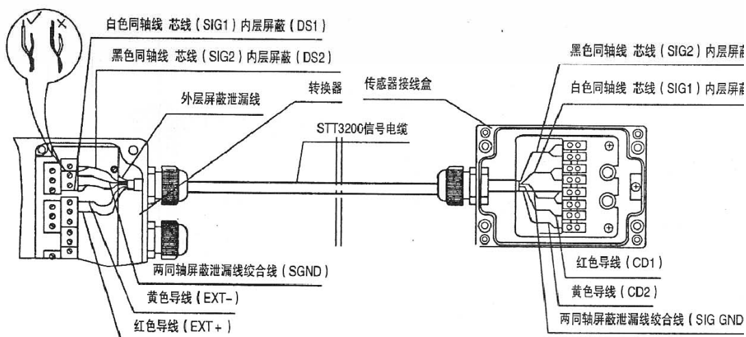
图十一 分离型传感器与转换器的连接
