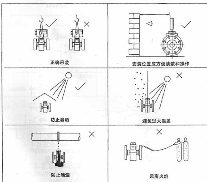
图六 正确安装流量计图示一
