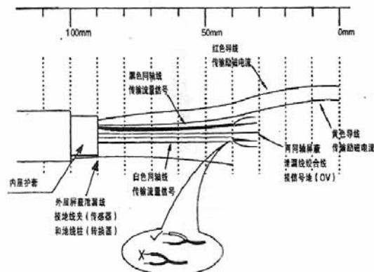
图十二 STT3200电缆剥线示意图
