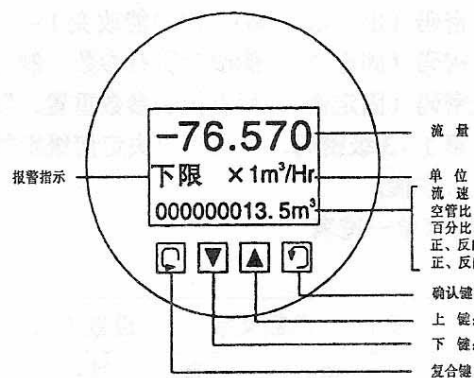
图五 (b) 圆表键盘
