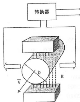
图一 电磁流量计工作原理
