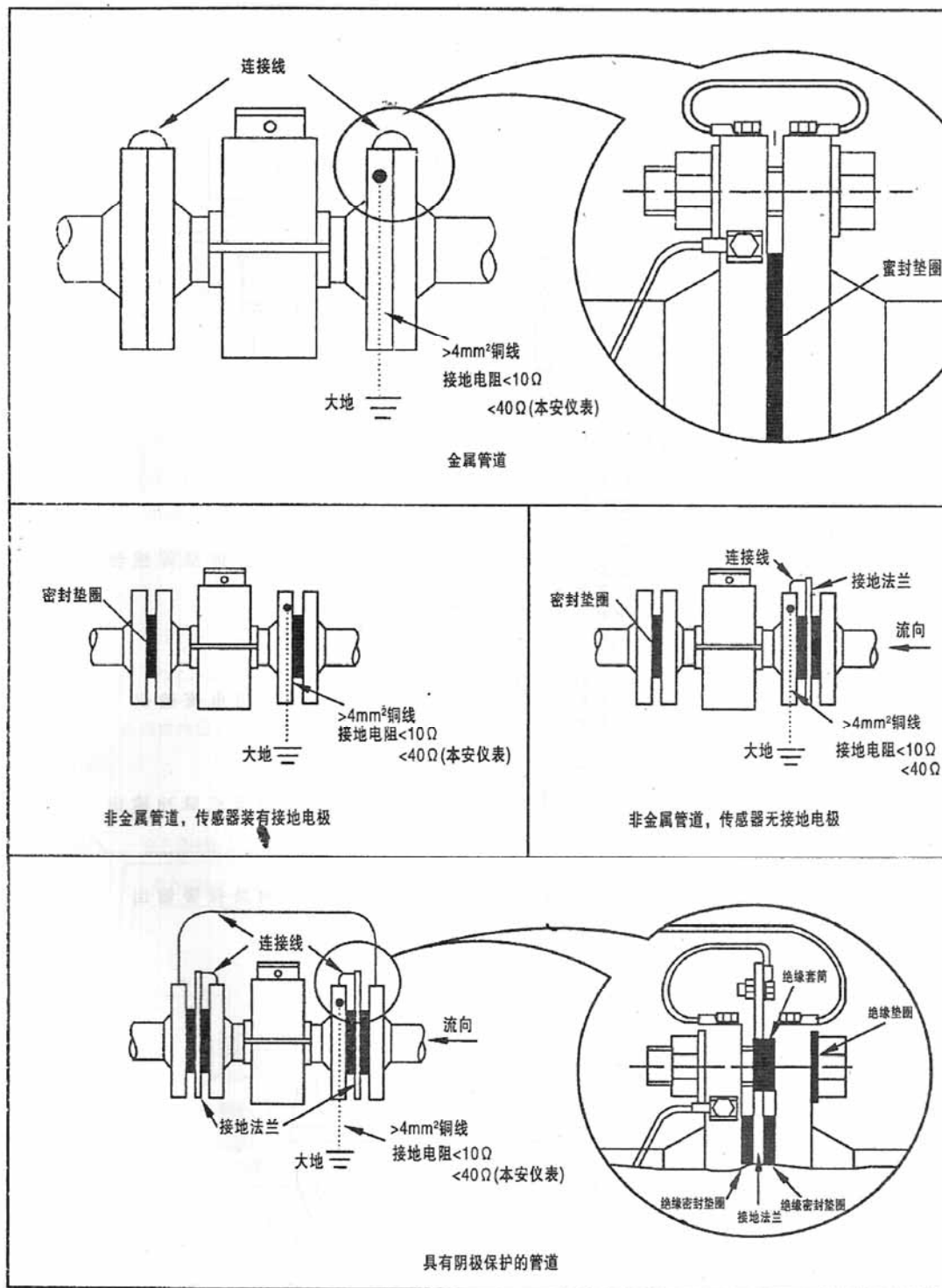
图七 流量计与管道的接地
