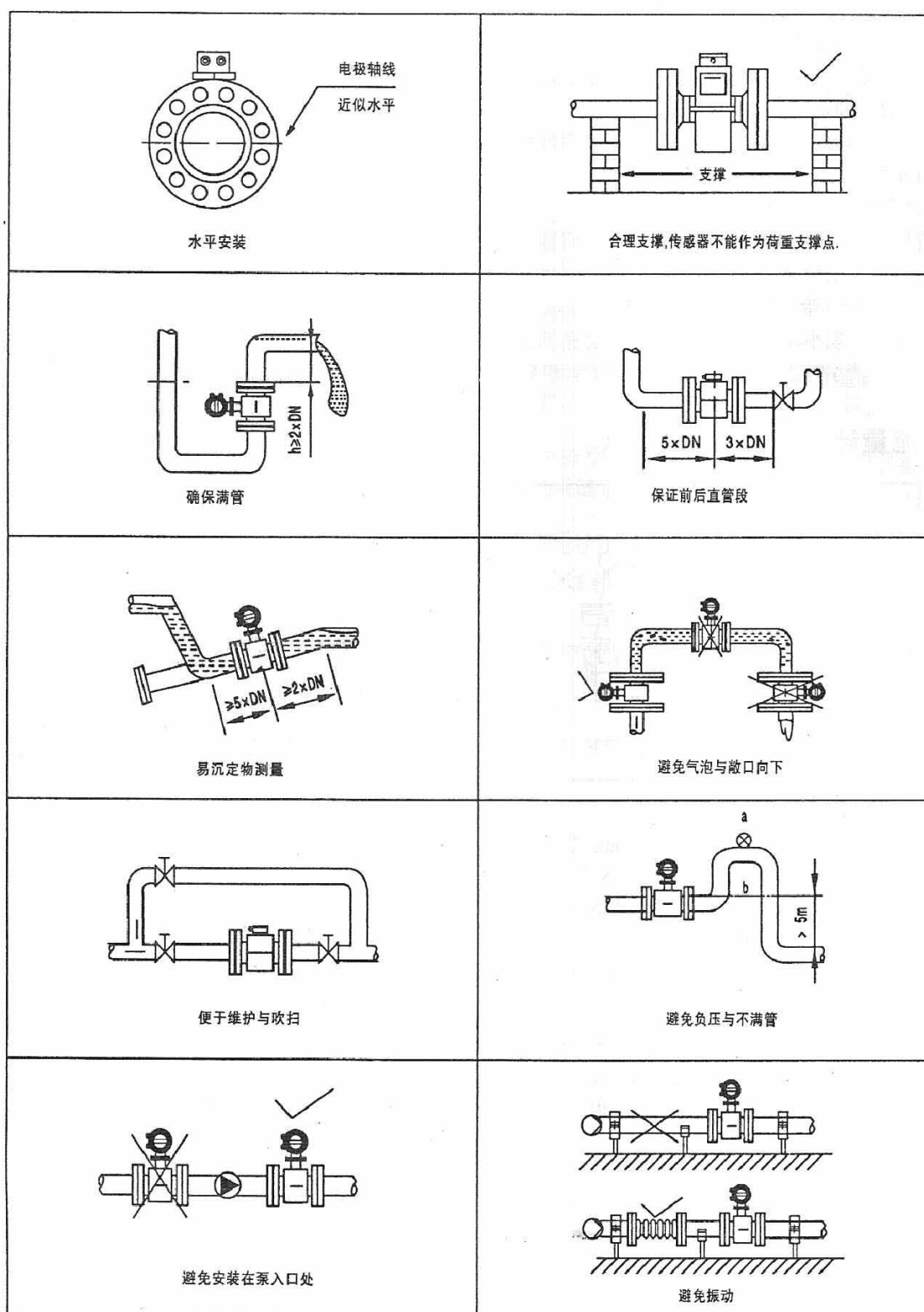
图六 正确安装流量计图示二
