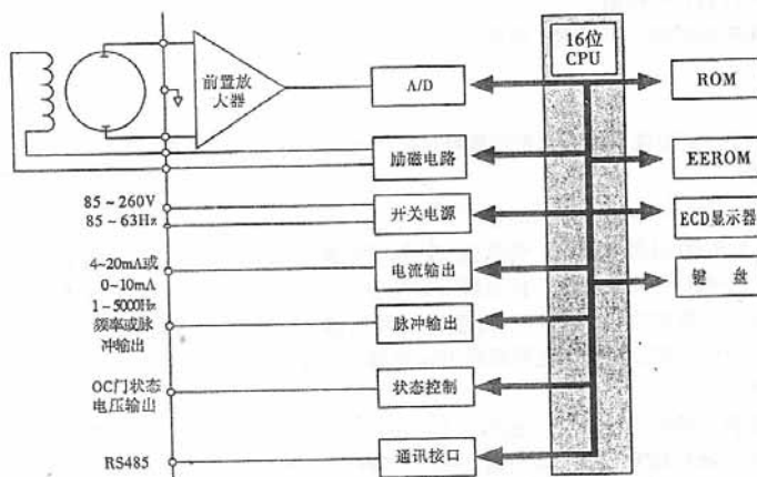
图二 转换器电路结构
