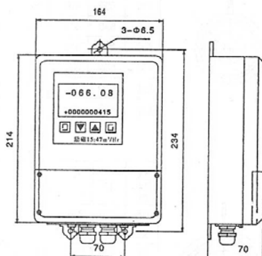
图三（b）方转换器外形
